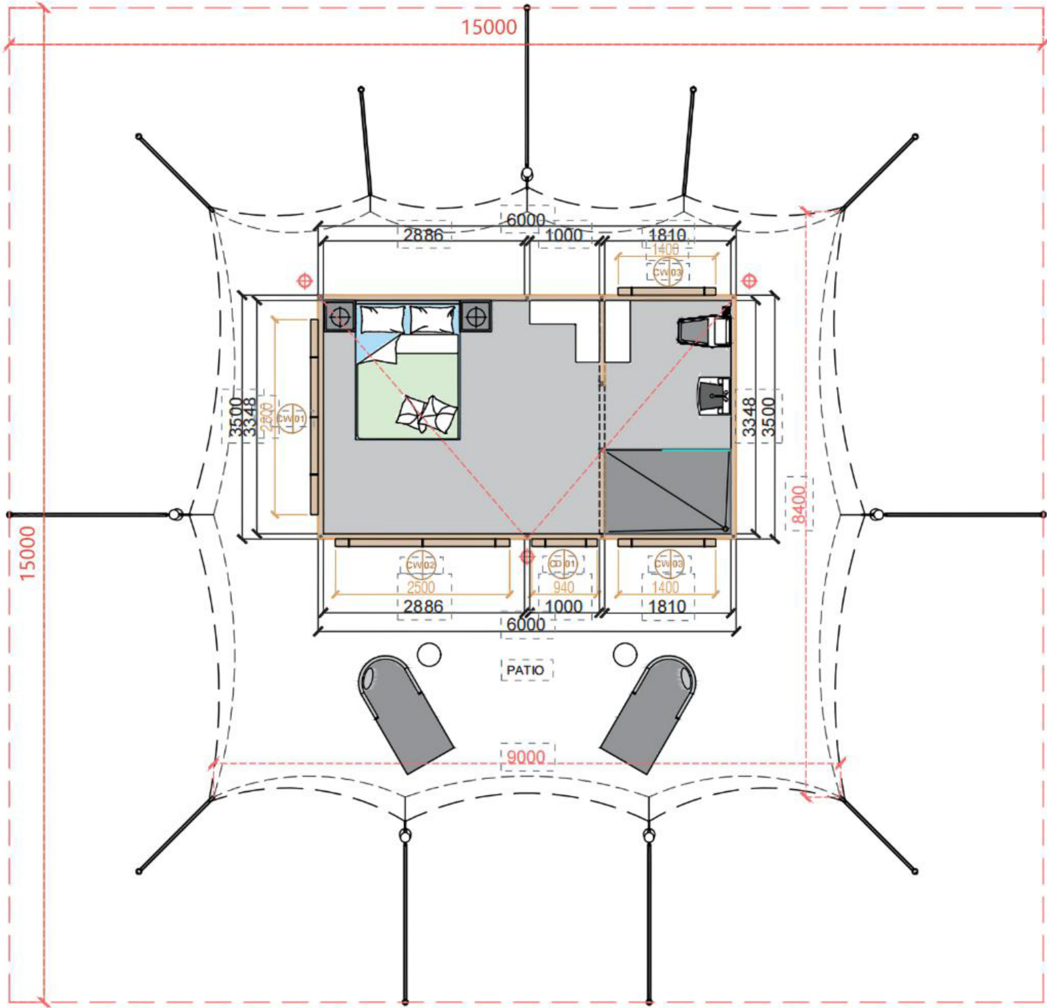
平面尺寸图
