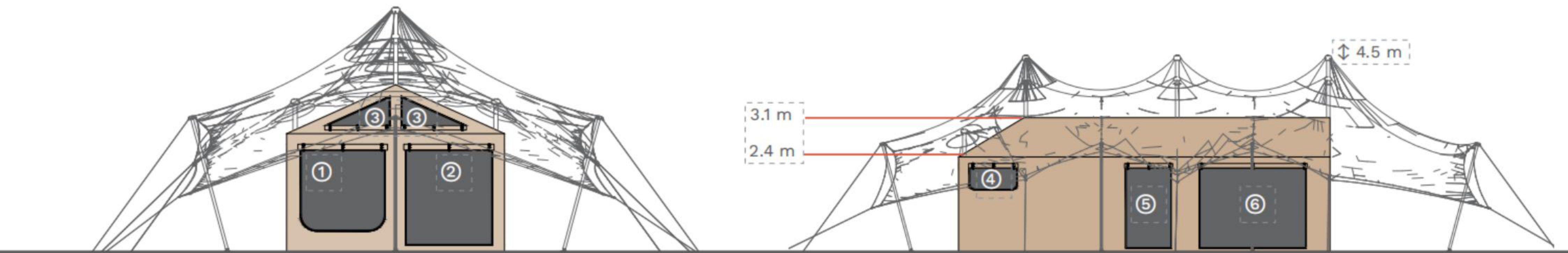
立面图
