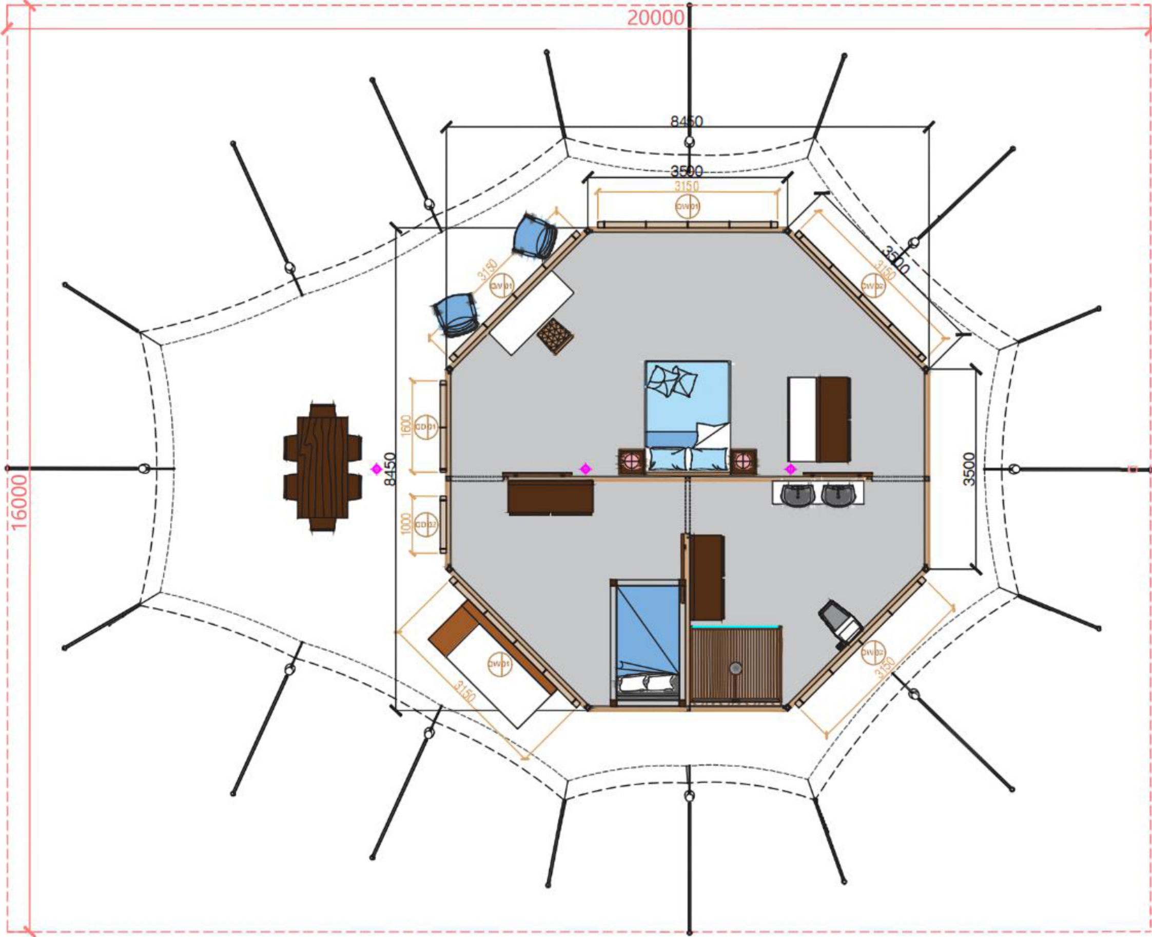
平面尺寸图
